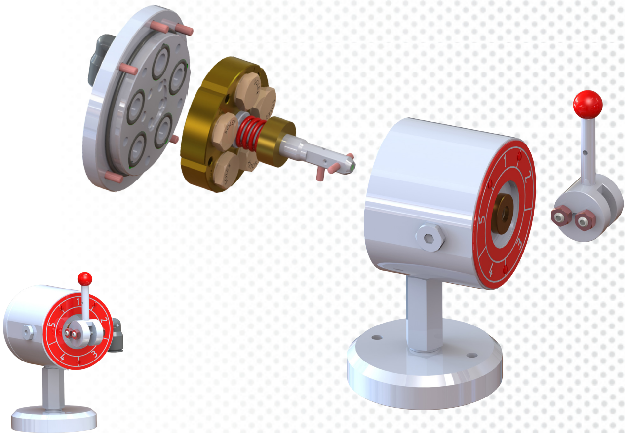
Barillet Multi-gigleurs
