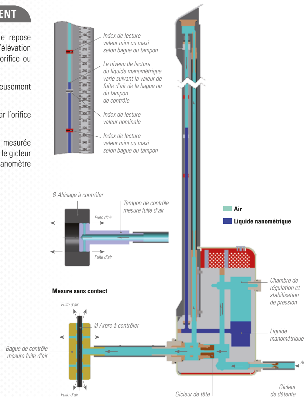
Schéma de principe fonctionnel du micromesureur pneumatique
